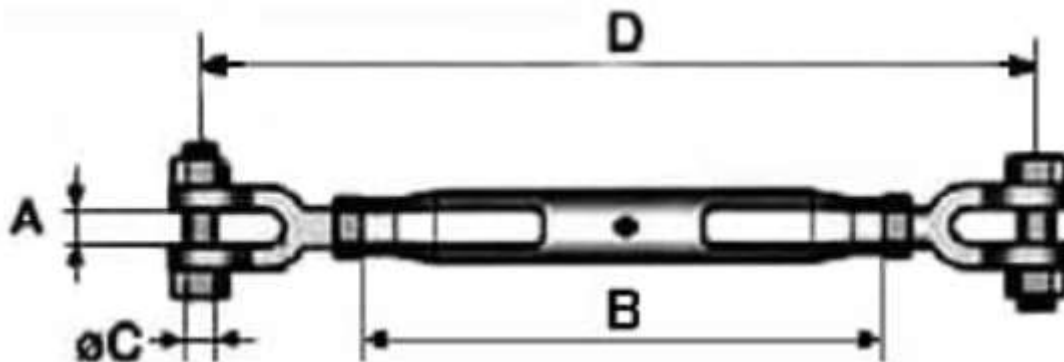
Рис.1 - Чертеж талрепа вилка-вилка (закрытого типа)
